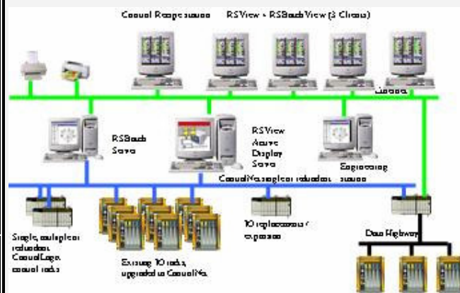
Hardware architectuur
